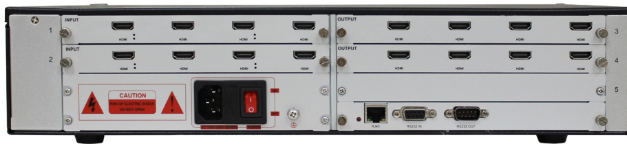
MXwall LT V2 (4x12) Front
